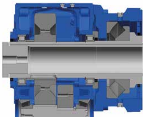
Esecuzione HA: estrazione della vite (con cava linguetta) sul lato opposto estrusore
