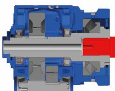
Spallamento a vite sul lato anteriore
