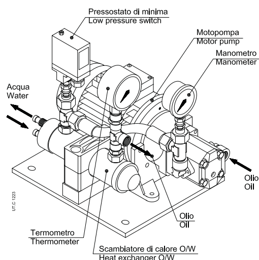
Cuscinetti estrusore con lubrificazione forzata tramite unità di raffreddamento esterna
