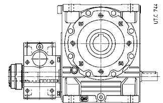
Montage du limiteur dans les groupes (combinés)
