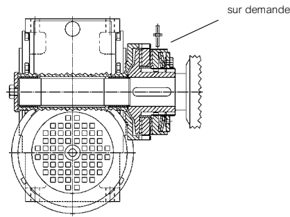
Montage du limiteur intermédiaire
