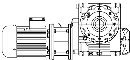
MLA montage entre réducteur et moteur ou motovariateur
