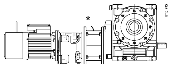
MLA montage dans les groupes (combinés)
