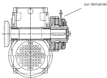
Montage du limiteur externe
